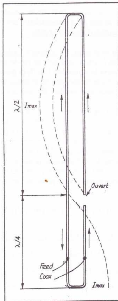
Fig. 3. — Fonctionnement de la Slim Jim.
