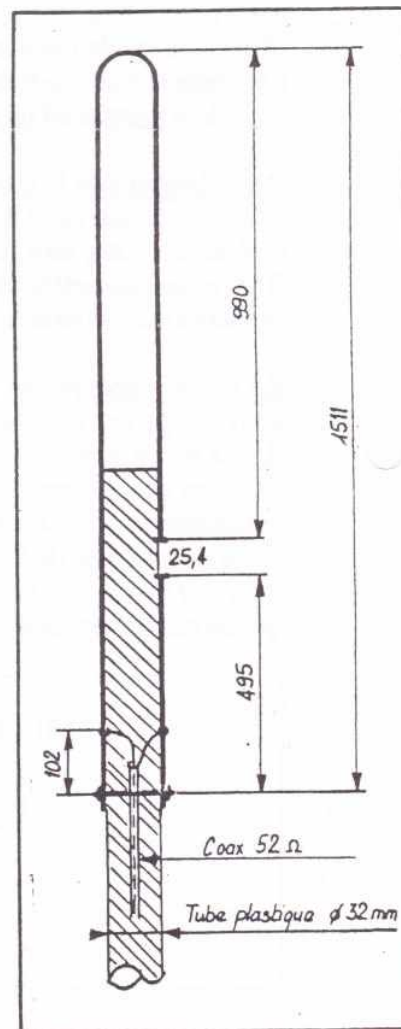
Fig. 4. — Réalisation de la Slim Jim.
